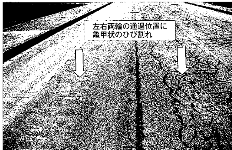
写真-1 アスファルト舗装の破損状況 (200 m 以上にわたり連続した破損)
